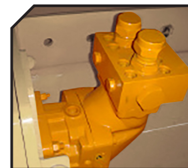
Válvula anti retorno incorporada no motor
